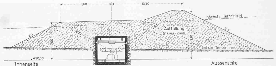
Bild 10. Magnetring des Proton-Synchrotrons, Querschnitt 1:400
